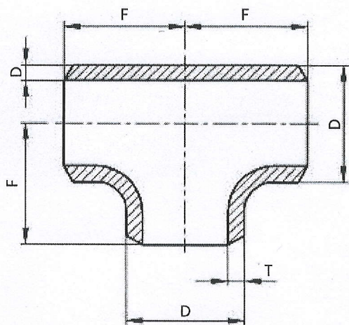
T-kusy se stejnými hrdly | T-pieces with equal throats Тройники с идентичными горлами
