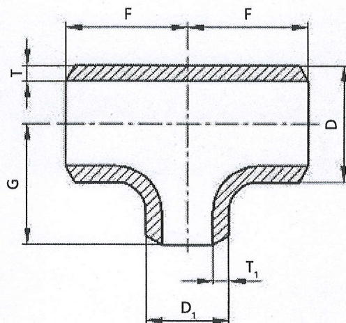
T-kusy s nesterými hrdly | T-pieces with unequal throats Тройники с неидентичными горлами
